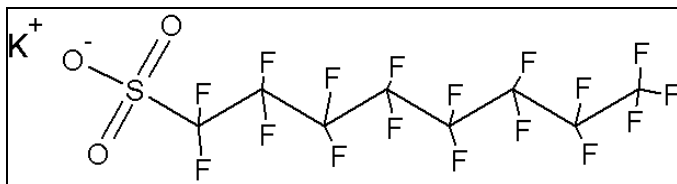
图 1. 图中显示是其钾盐的结构式
