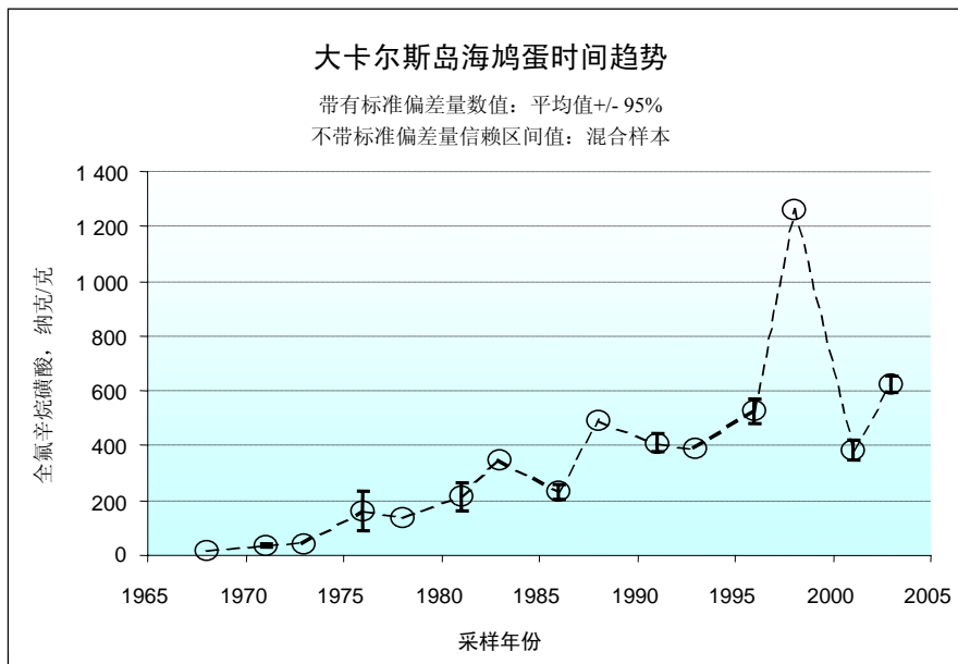
图 2. 1968-2003 年在波罗的海大卡尔斯岛采集的海鸬 ( Uria aalge ) 蛋中测得的全氟辛烷磺酸浓度。该图表来自瑞典环境保护署环境评估部 “Screening av perfluorerade ämnen” 报告 (2004 年)
